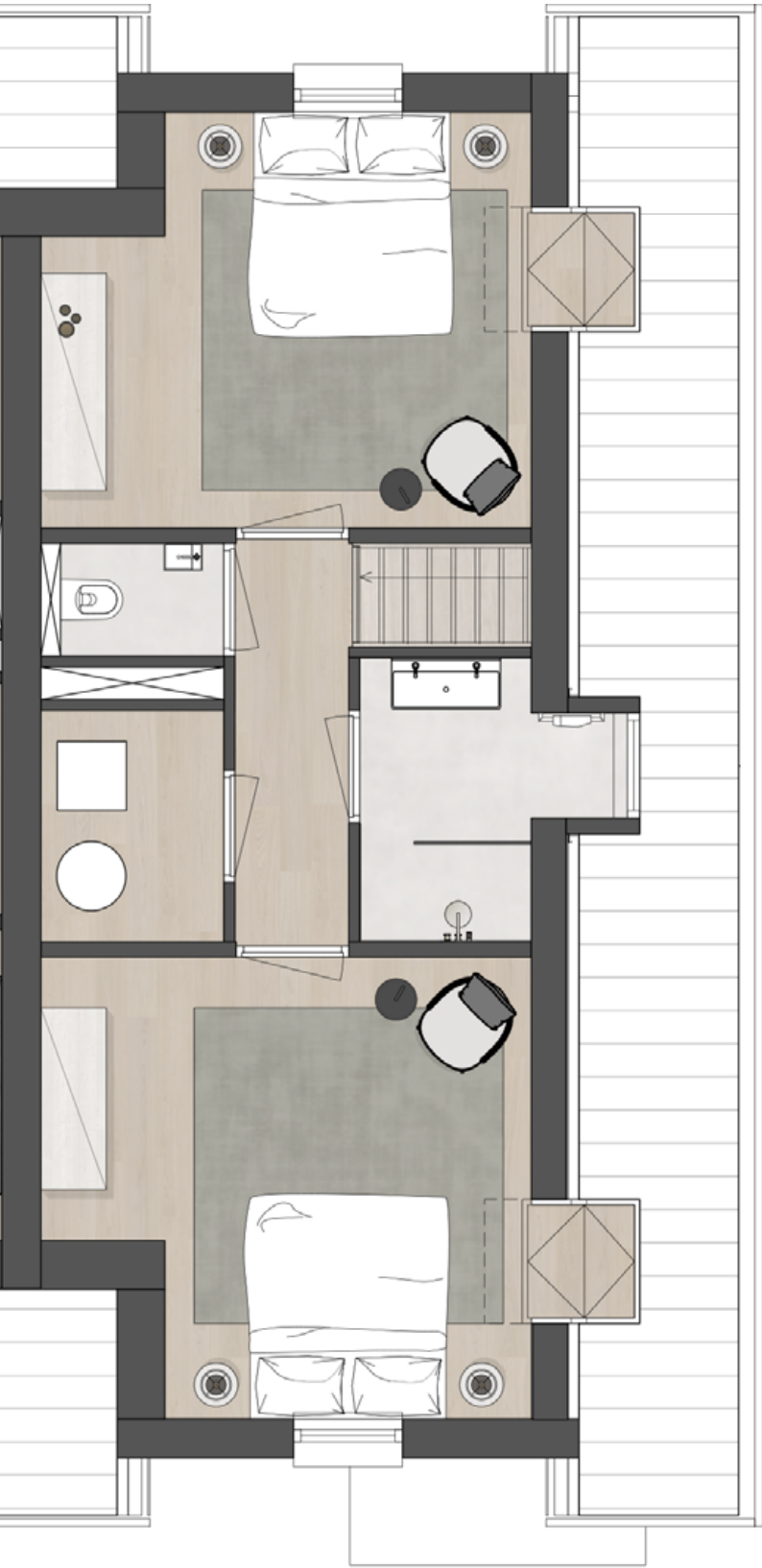
2e verdieping
